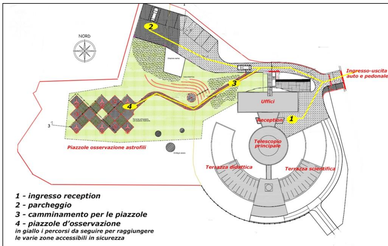
Fig. 3. Pianta dell'Osservatorio Astronomico (gennaio 2014). In giallo sono indicati i percorsi che è obbligatorio seguire per raggiungere in sicurezza la nuova area di osservazione allestita nella parte occidentale della struttura, con le piazzole prenotabili da astrofili e appassionati.
